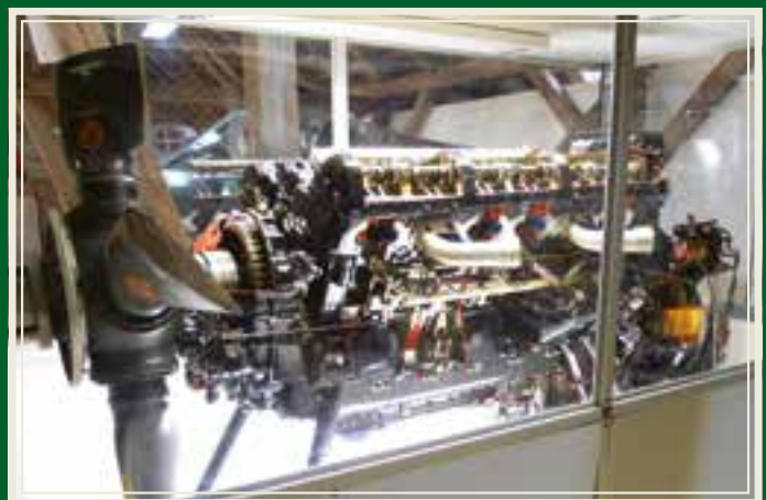
Oppskåret Rolls-Royce Merlin 70, v12 flymotor med 27 liter slagvolum og 1250 hp, brukt i Supermarine Spitfire HF Mk.VIII, HF.IX og PR.XI.
